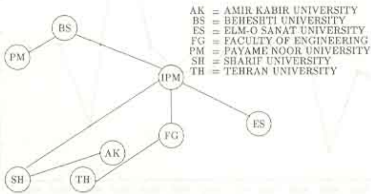
نحوه اتصال دانشگاههای داخل تهران (این طرح با موافقت شرکت مخابرات تهیه گردیده و قابل تحمیر است).
